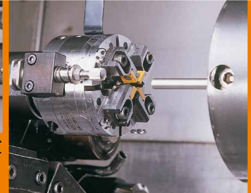
MSD 20-R, obrotowa ▲
